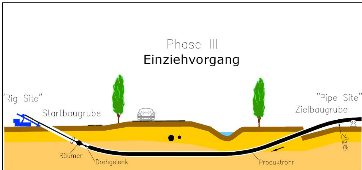
Abbildung 1.7-3: HDD-Verfahren Phase III – Einziehvorgang
