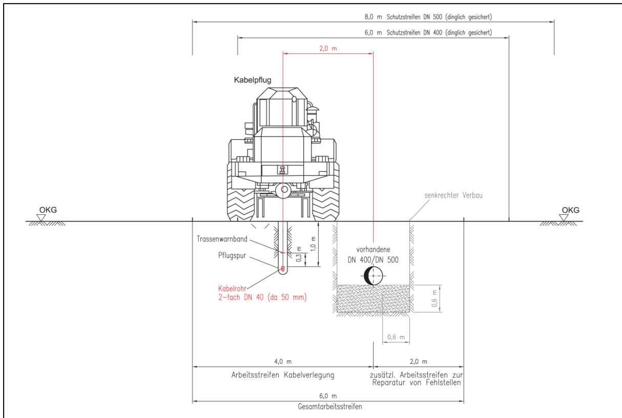
Abbildung 1.7-2: Arbeitsstreifen für Kabelverlegung parallel zur vorhandenen FGL 012
