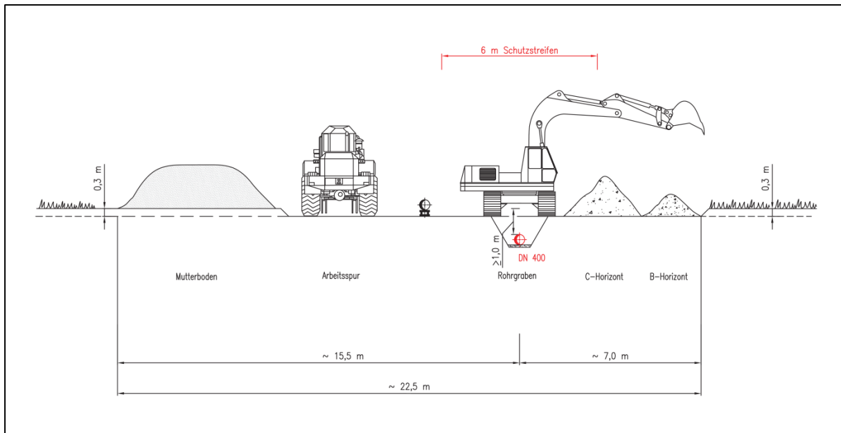
Abbildung 1.7-1: Regelarbeitsstreifen DN 400 im Offenland
