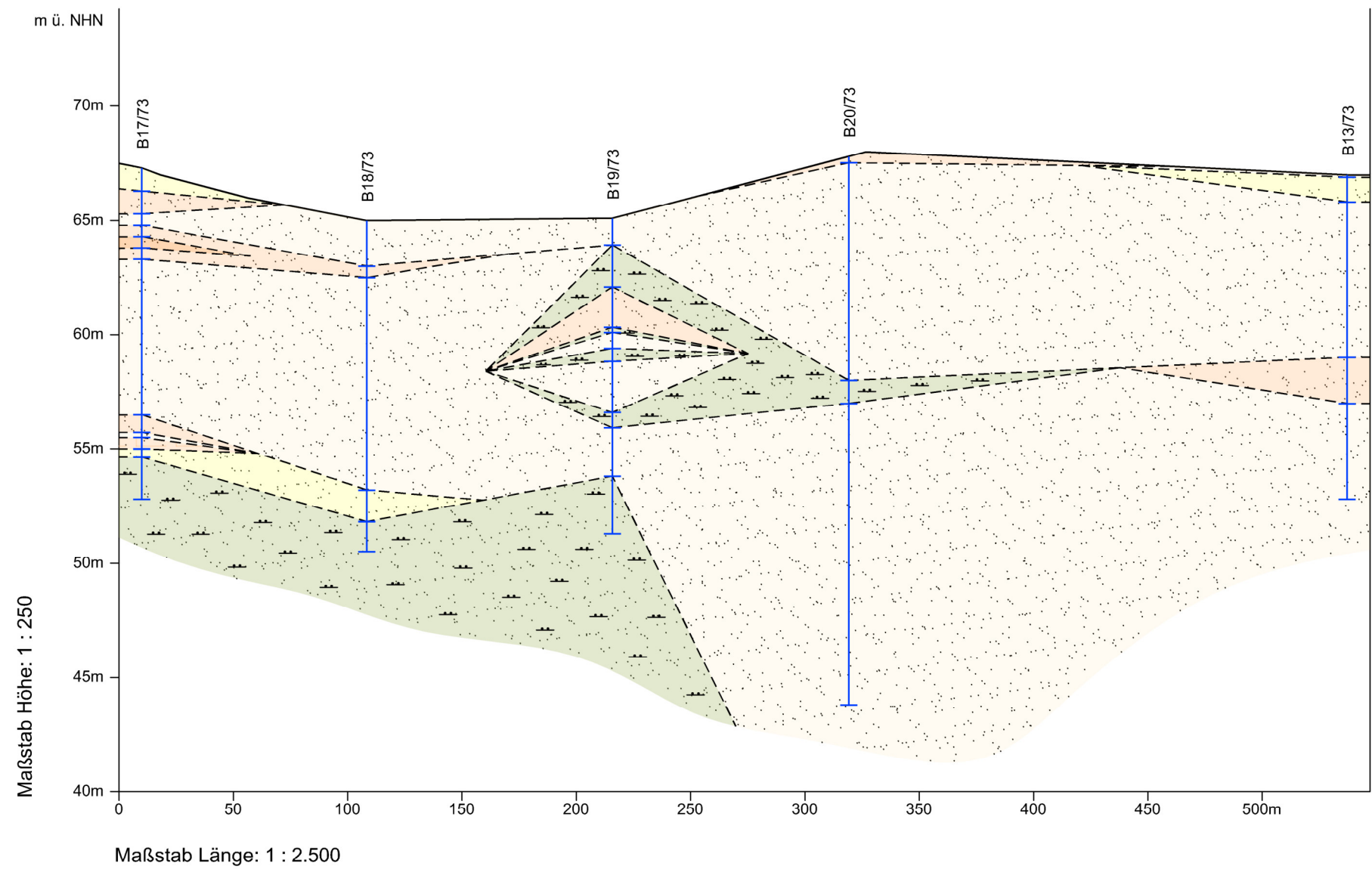
Schematische Schnittdarstellung A - A'
