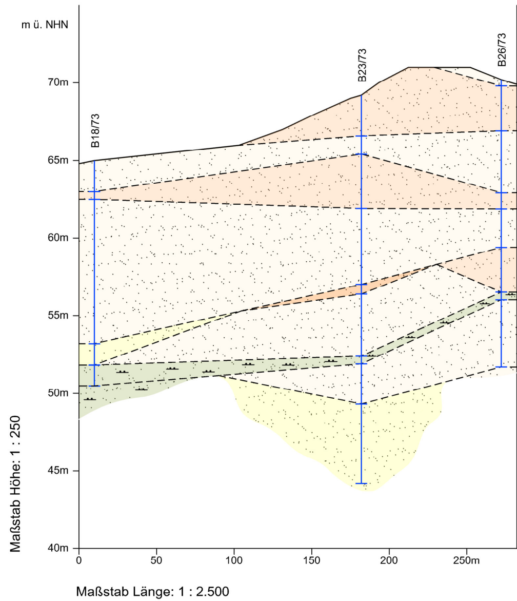
Schematische Schnittdarstellung B - B'
