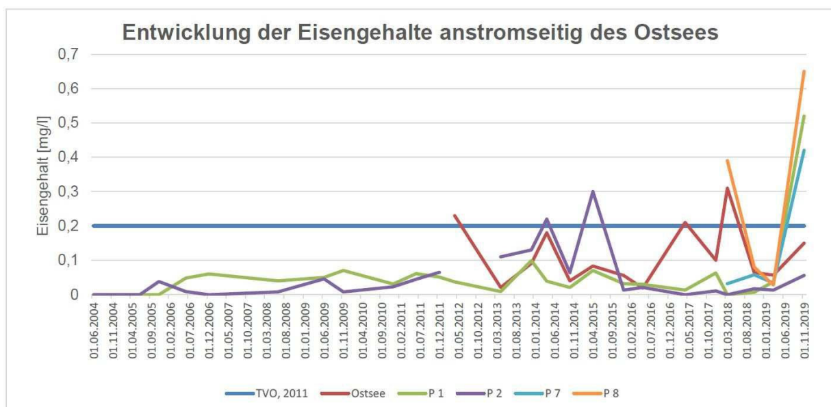
Abb. 1413: Entwicklung der Eisengehalte anstromseitig des Ostsees 2004 - 2019 (G.E.O.S. 2020b)
