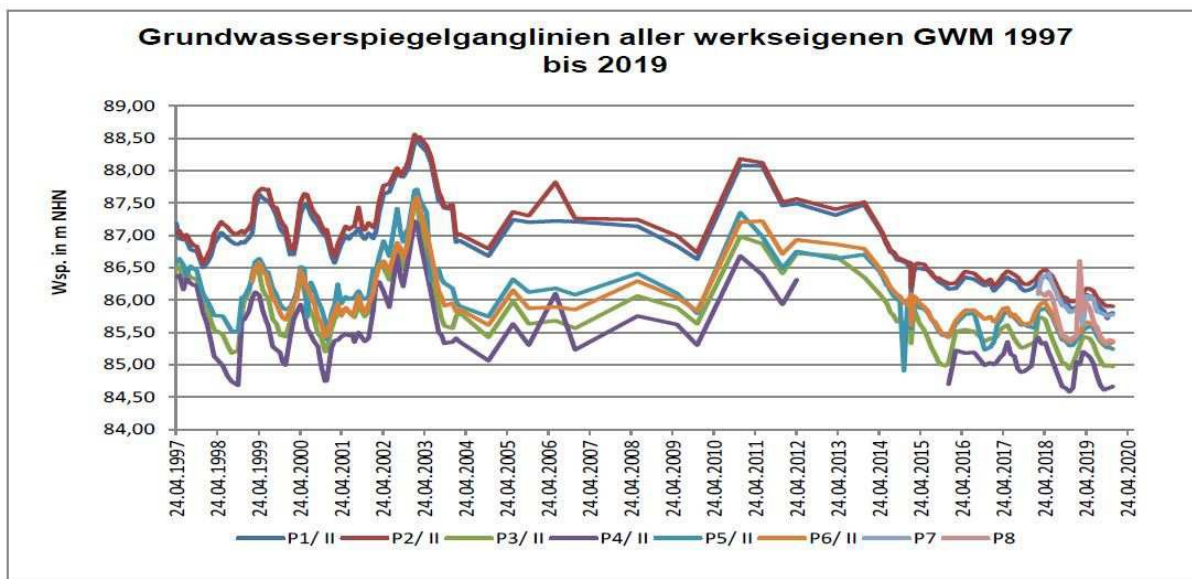
Abb. 98: Grundwasserspiegelganglinien der Werks-GWM im Zeitraum April 1997 – Januar 2020 (aus G.E.O.S 2020a)
