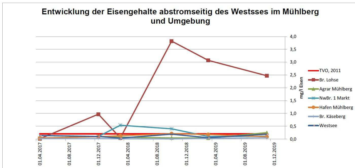
Abb. 4514: Entwicklung der Eisengehalte abstromseitig des Westssee in Mühlberg und Umgebung 2017 - 2019 (G.E.O.S. 2020b)
