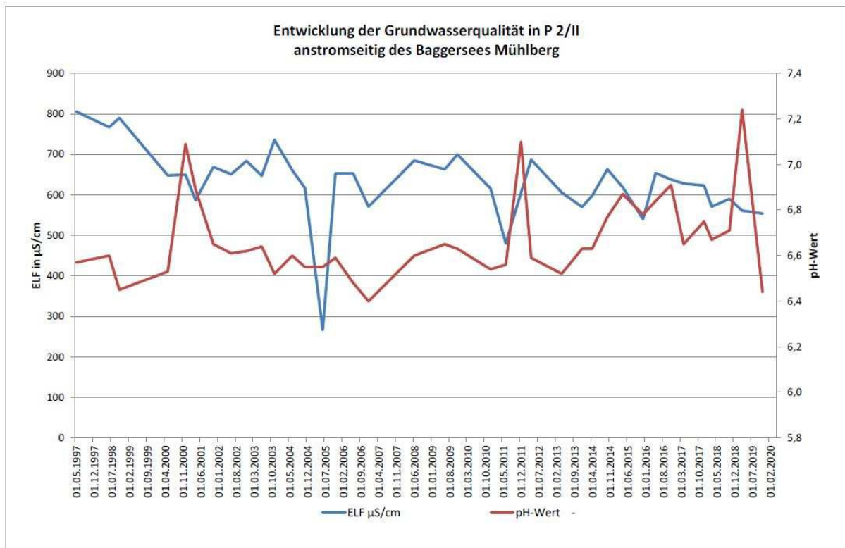
Abb. 409: Entwicklung der elektrischen Leitfähigkeit und des pH-Wertes anstromseitig des Baggersees OT Weinberge von 1997 – 2020 (G.E.O.S. 2020b)
