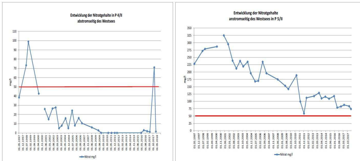
Abb. 4312: Nitratgehalte im Zeitraum 1997 - 2020 abstromseitig des Westsees (G.E.O.S. 2020b)
