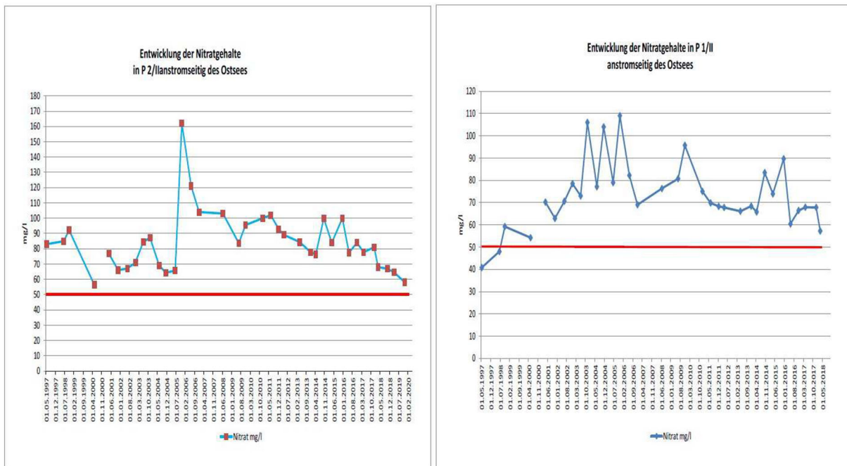
Abb. 4211: Nitratgehalte im Zeitraum 1997-2020 anstromseitig des Ostsees (aus G.E.O.S. 2020b)
