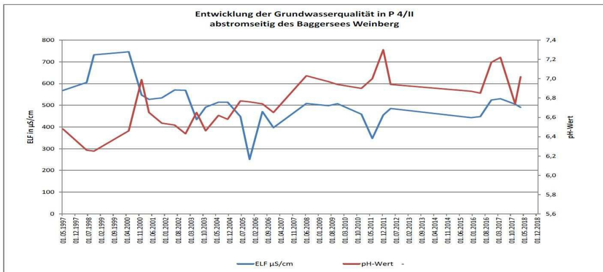
Abb. 4410: Entwicklung der elektrischen Leitfähigkeit und des pH-Wertes abstromseitig des Baggersees Mühlberg von 1997 – 2020 (G.E.O.S. 2020b)
