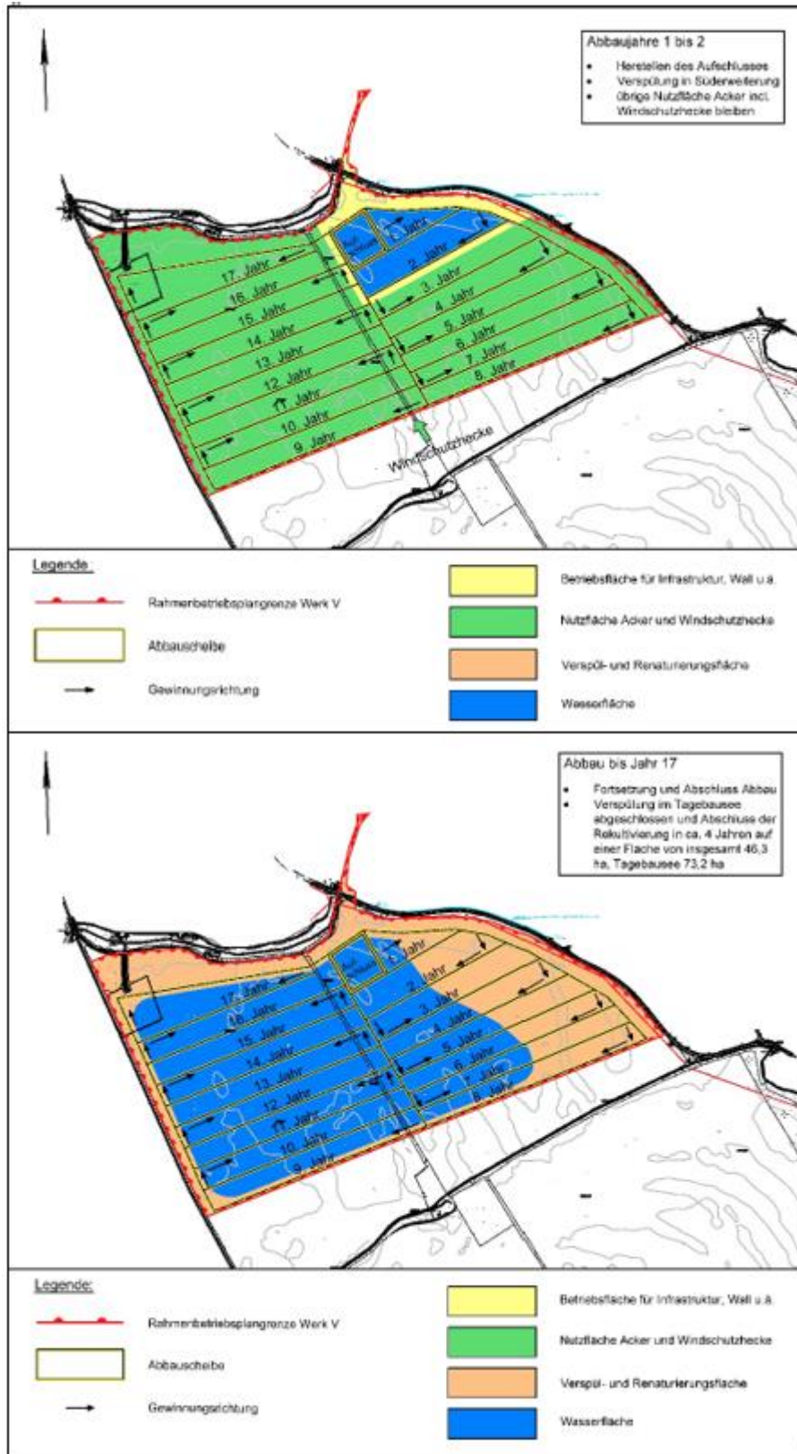
Abbildung 4 Vorhabenplanung Tagebau Mühlberg, Werk V, Beginn und Ende des Abbaus sowie Verspölung /14/
