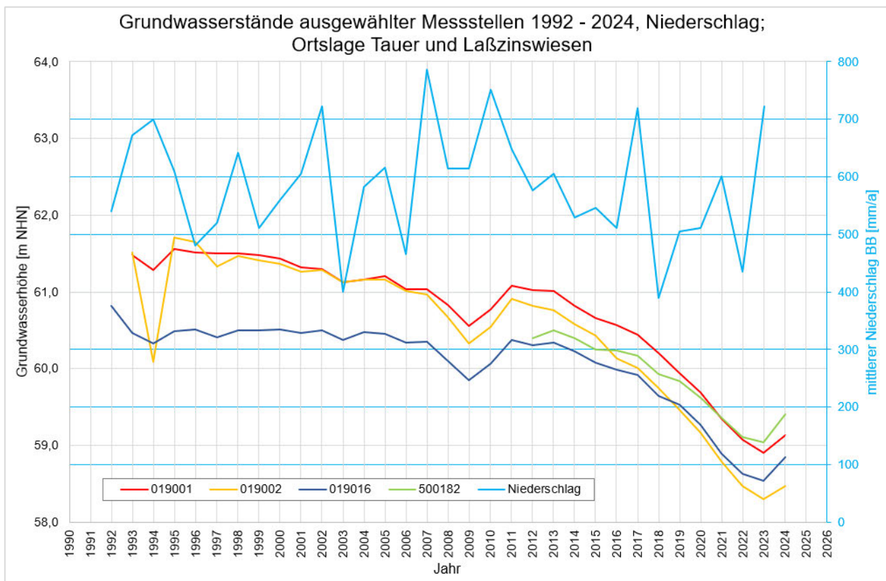
Abbildung 4: Grundwasserhöhen im Untersuchungsbereich Tauer und Niederschläge 1992 - 2024
