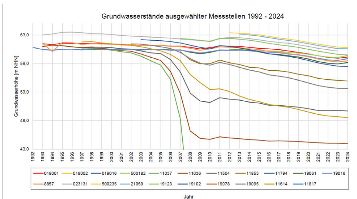
Abbildung 6: Entwicklung der Grundwasserstände im Zeitraum 1992 bis 2024
