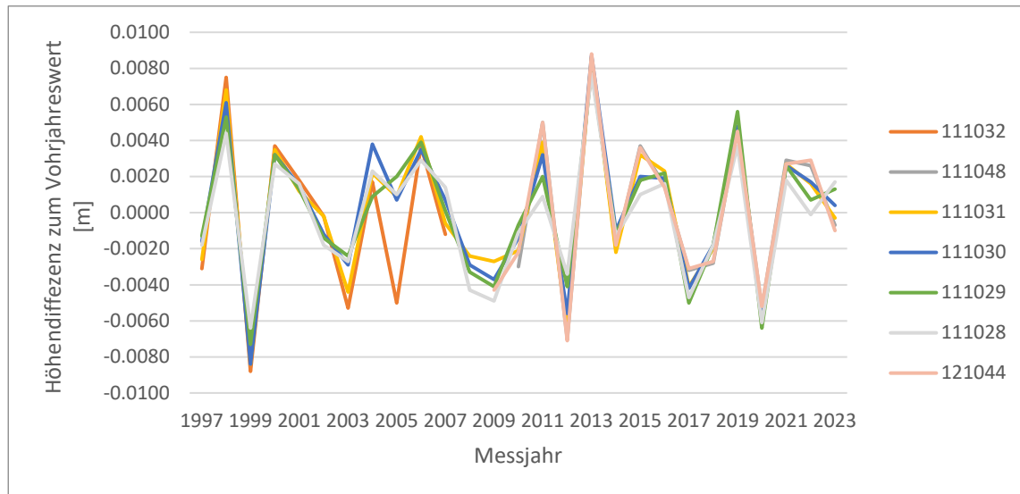
Abbildung 5: Höhendifferenz der Messdaten zum jeweiligen Vorjahreswert
