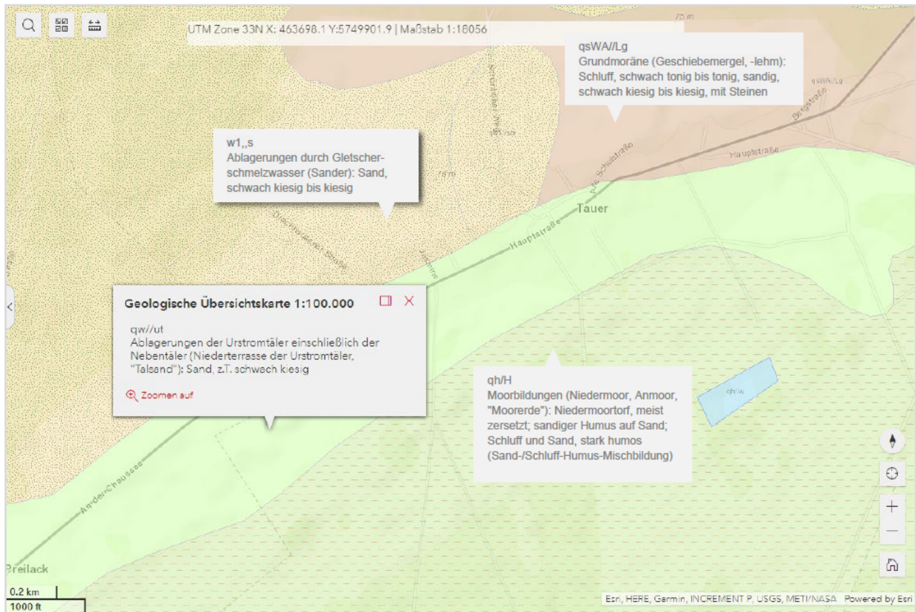
Abbildung 1: Auszug aus der geologischen Übersichtskarte 1:100.000 (Stand 2005 – 2015) Untersuchungsbereich Ortschaft Tauer; aus [11]
