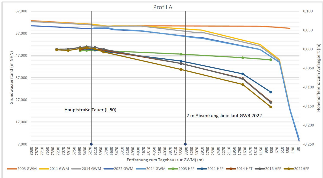
Abbildung 8: Gegenüberstellung der entfernungsabhängigen Grundwasserstände und Höhendifferenzen für das Profil A mit Markierung der 2-m-Absenkungslinie (LEAG) und der Hauptstraße von Tauer/Landesstraße L 50 (aus Anlage 4)
