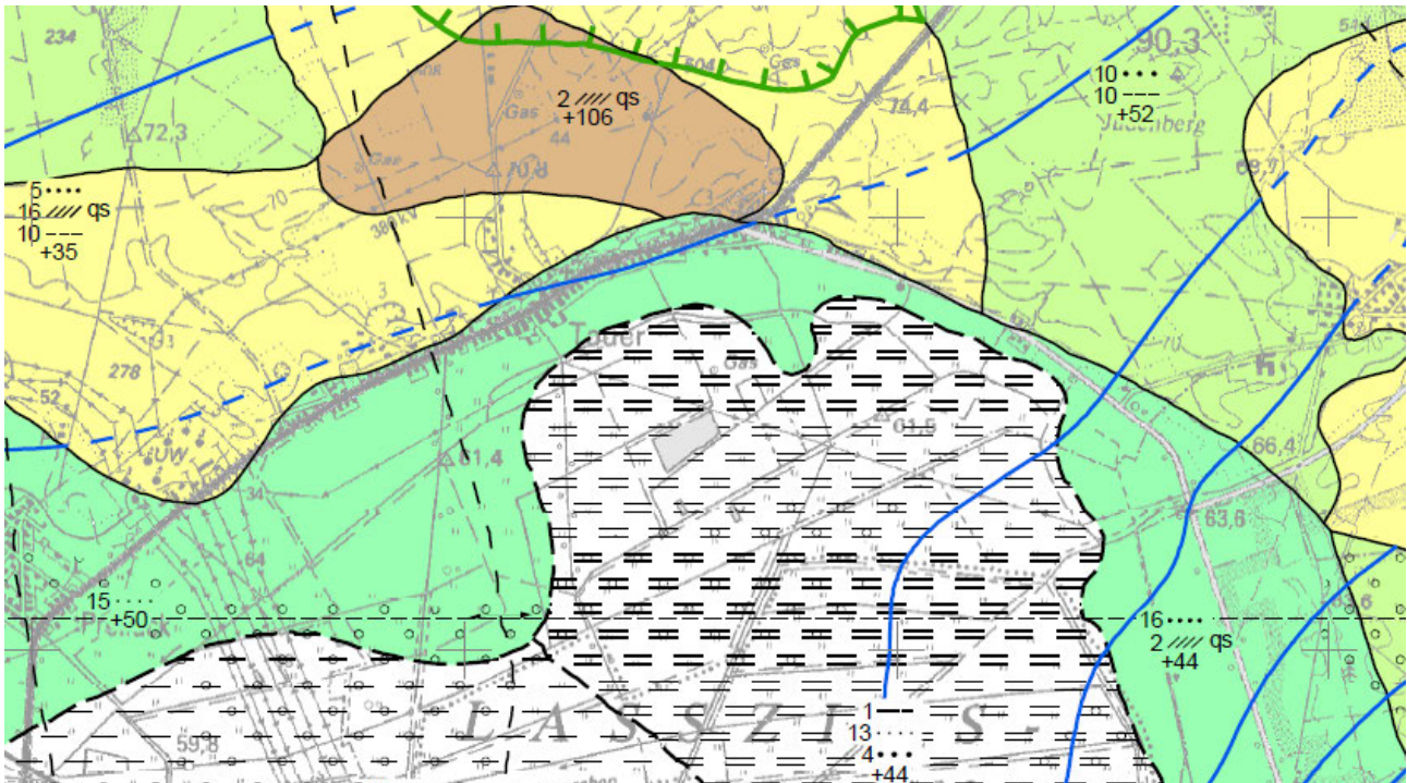
Abbildung 2: Ausbildung des GWLK 1 in Tauer und Umgebung; weiß: Torf, grün: unbedeckter Grundwasserleiter, gelb: trockene Sande, braun: Geschiebemergel und -lehm; aus [8]
