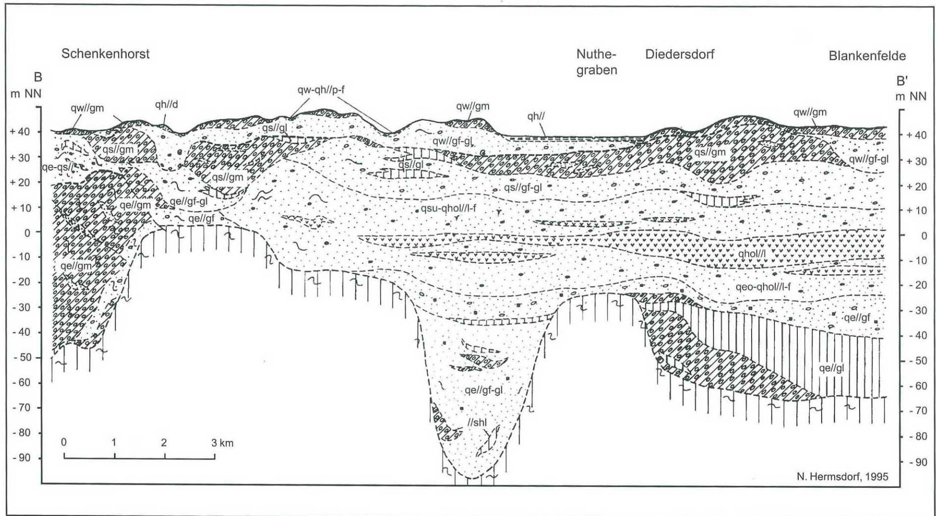
Abb. 4 Geologischer Schnitt (E-W - Profil) durch den Westteil des Teltows (Legende wie Abb. 3)
