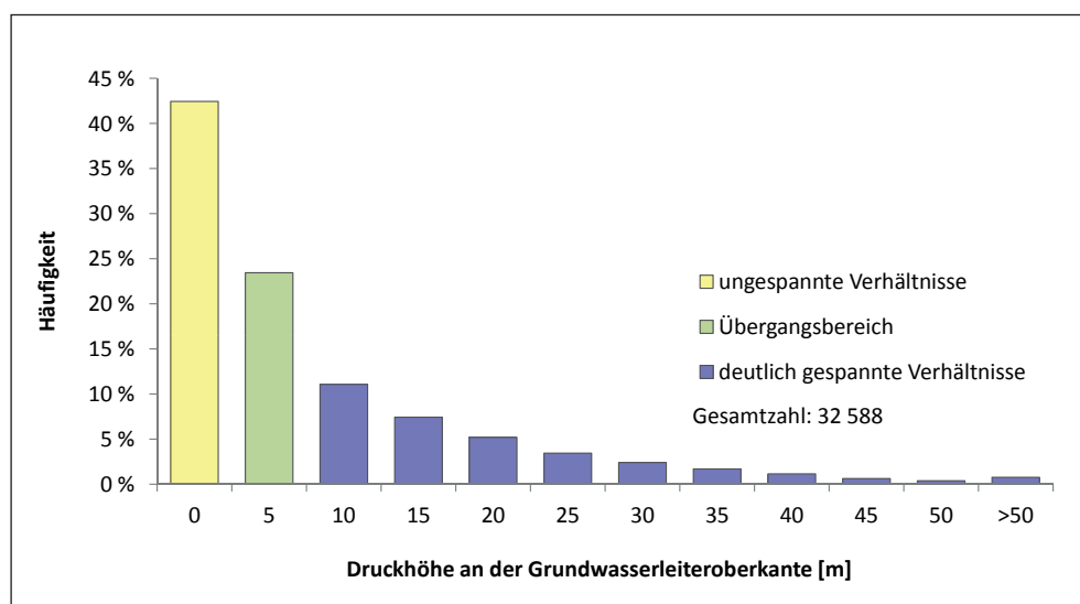
Abb. 1: Häufigkeitsverteilung der Druckhöhe an der Grundwasserleiteroberkante (Auswertung der im Landesbohrdatenspeicher Mecklenburg-Vorpommern erfassten Aufschlüsse)
