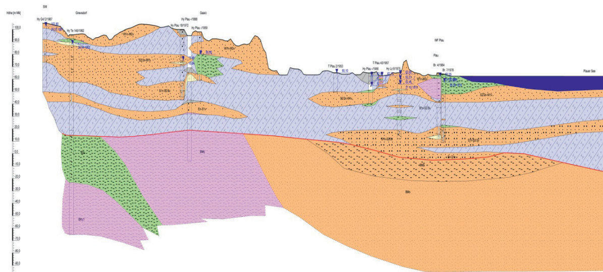
Abb. 5: Hydrogeologische Profilschnitte – Beispiele für die Grundwasserspeisungstypen 1, 2 und 3 Fig. 5: Hydrogeological profile sections – examples of groundwater infiltration types 1, 2 and 3
