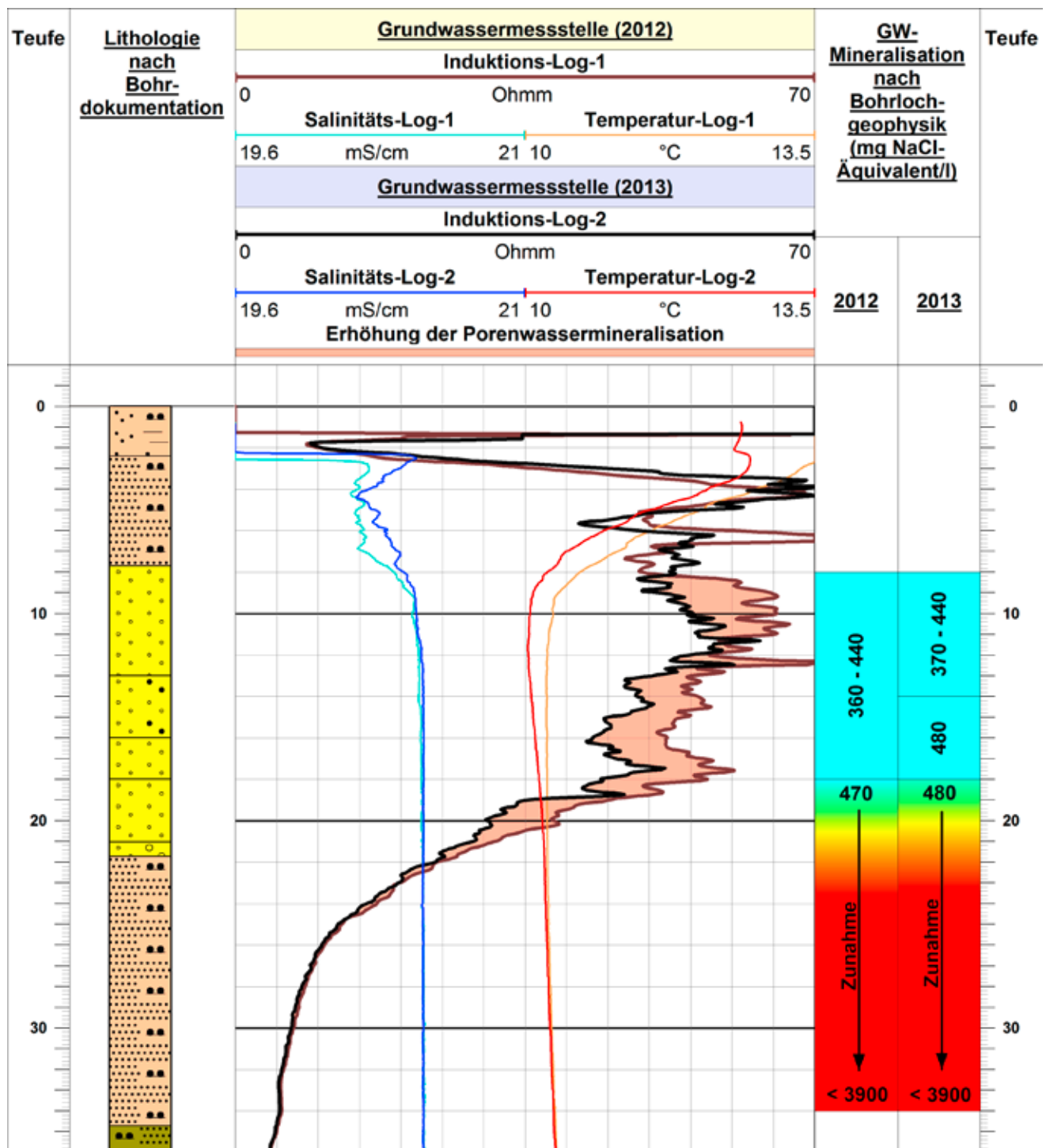
Abb. 5: Erhöhung der Porenwassermineralisation im oberen Grundwasserleiter in der Grundwassermessstelle in Lenz (Elbe)
