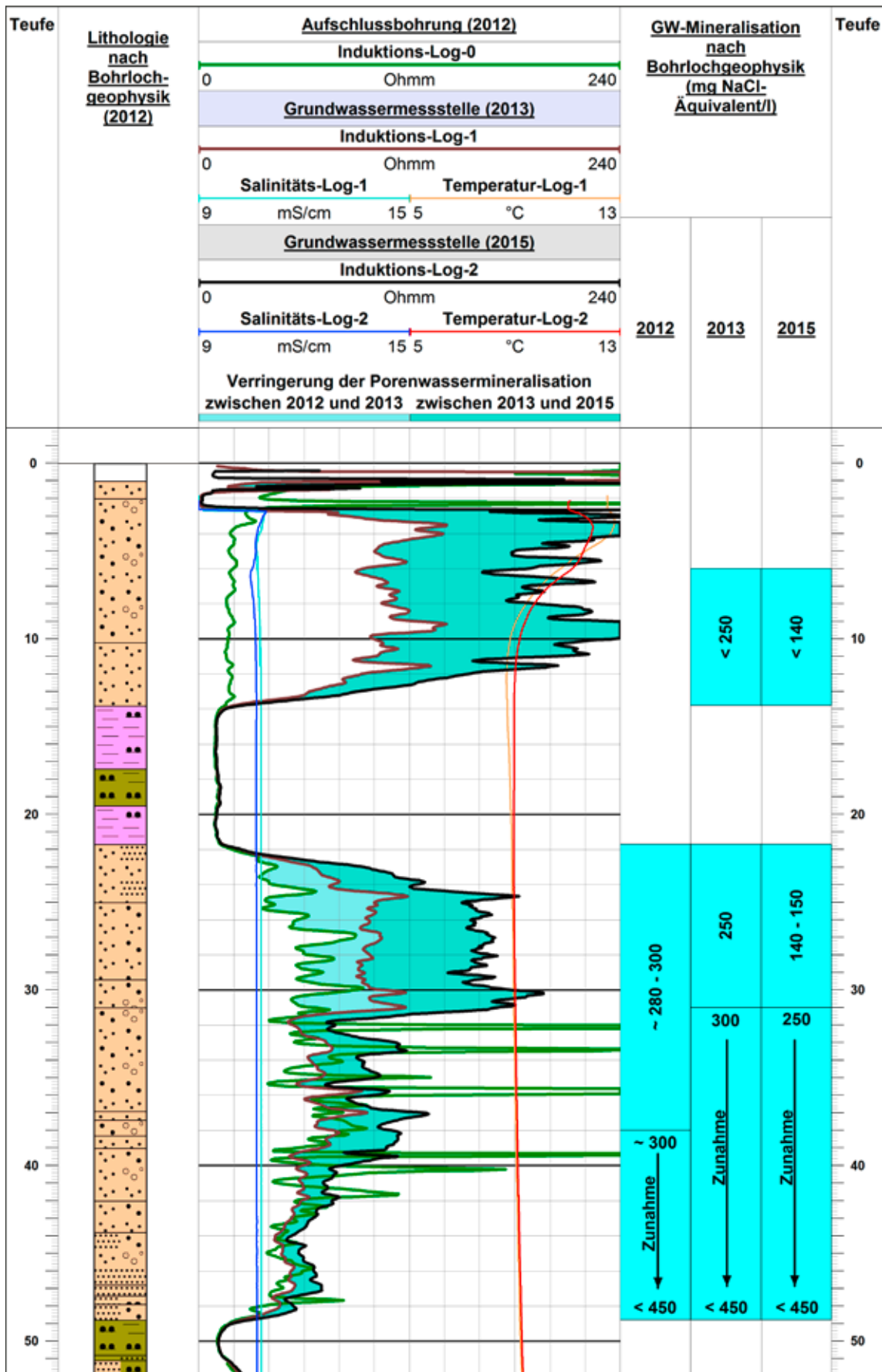
Abb. 6: Verringerung der Grundwassermineralisation in der Grundwassermessstelle in Biegenbrück
