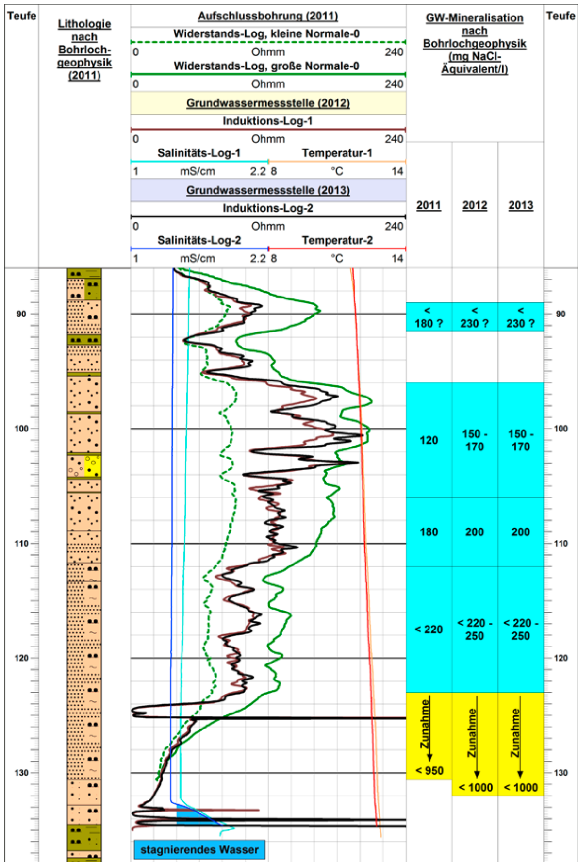
Abb. 7: Unveränderte Porenwassermineralisation in der Grundwassermessstelle in Spreenhagen
