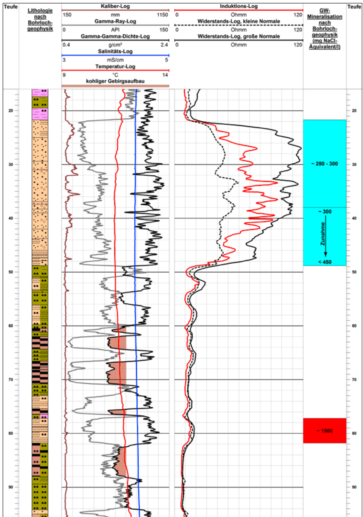
Abb. 2: Aufschlussmessung mit „Hydro-Standardprogramm“ im offenen Bohrloch
