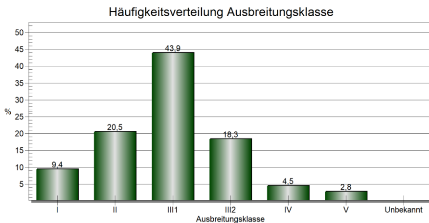
Abbildung 4. Häufigkeitsverteilung der Ausbreitungsklassen der DWD-Station Cottbus 2015
