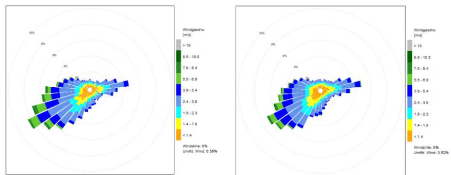
Windverteilung in Prozent 2015
