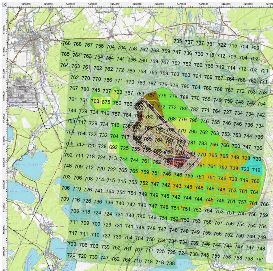
Abbildung 7. Regenverteilung im Untersuchungsgebiet, Cottbus 2015.
