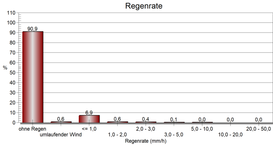
Abbildung 6. Regenstatistik für die DWD-Station Cottbus 2015, TB Jänschwalde.
