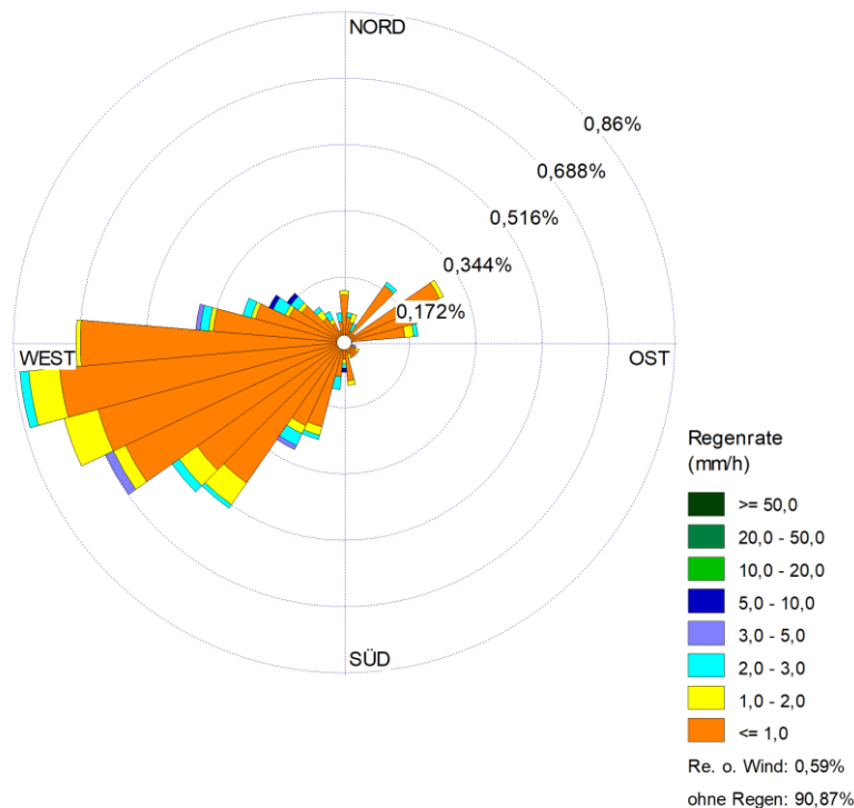
Abbildung 5. Windrichtungsverteilung der Regenrate, DWD-Station Cottbus 2015, TB Jänschwalde.
