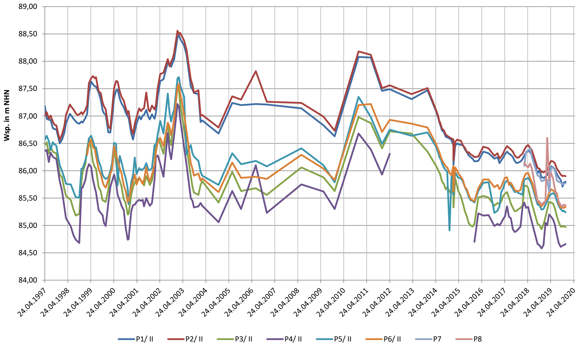
Grundwasserspiegelganglinien aller werkseigenen GWM 1997 bis 2019
